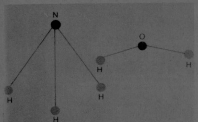
Molécula del amoníaco.
